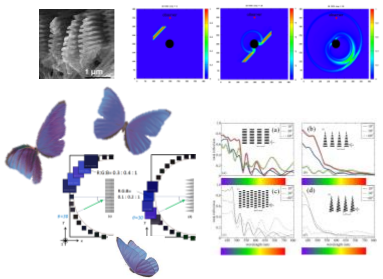
Fig.1 電磁波の基礎方程式から構造色を解析(FDTD法) 鱗粉のSEM像と電磁波の伝搬(上段)。入射・射出方向と鱗粉のモデルによる反射スペクトルの違い(下段)
